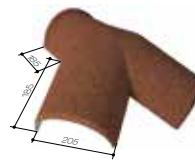
TRÓJNIK GAŚSIORA 205 30-45°
