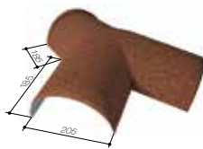
TRÓJNIK GAŚSIORA 205 15-30°
